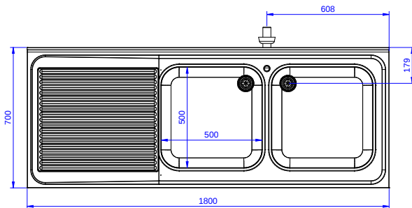
Boven aanzicht
