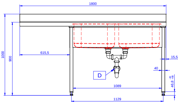
Zij aanzicht
